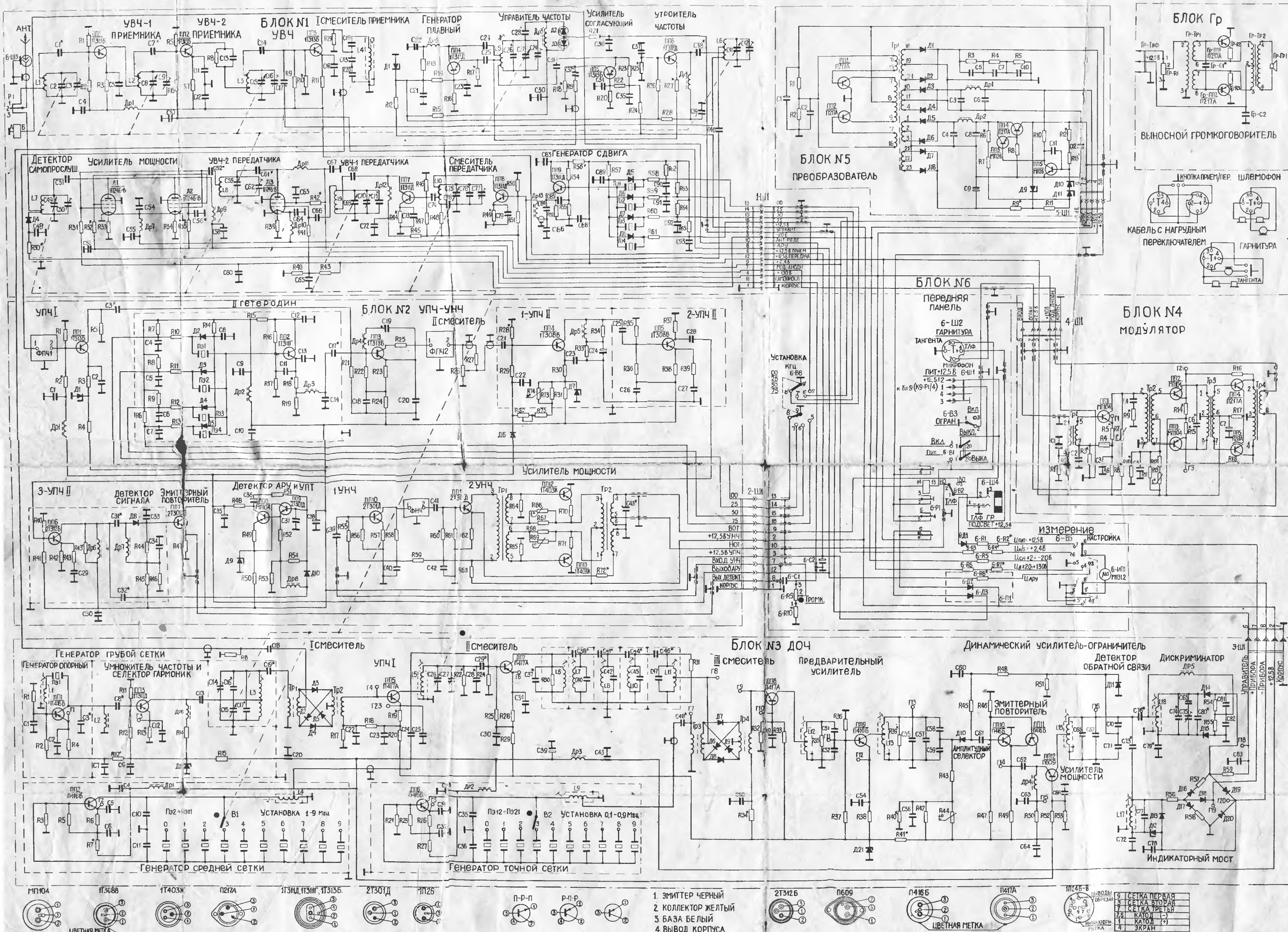
Принципиальная схема радиостанции Р-300М2.
